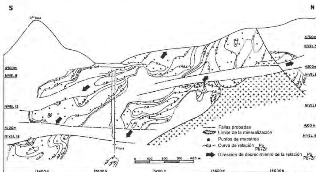
FIG. 2. Perfil longitudinal de la mina El Aguilar, 2.200 m en sentido norte-sur por 860 m de labores en profundidad, que muestra las curvas geoquímicas de isovalores para la relación Pb/Pb+Zn , con los límites de los cuerpos de mena y los puntos de muestreo.
