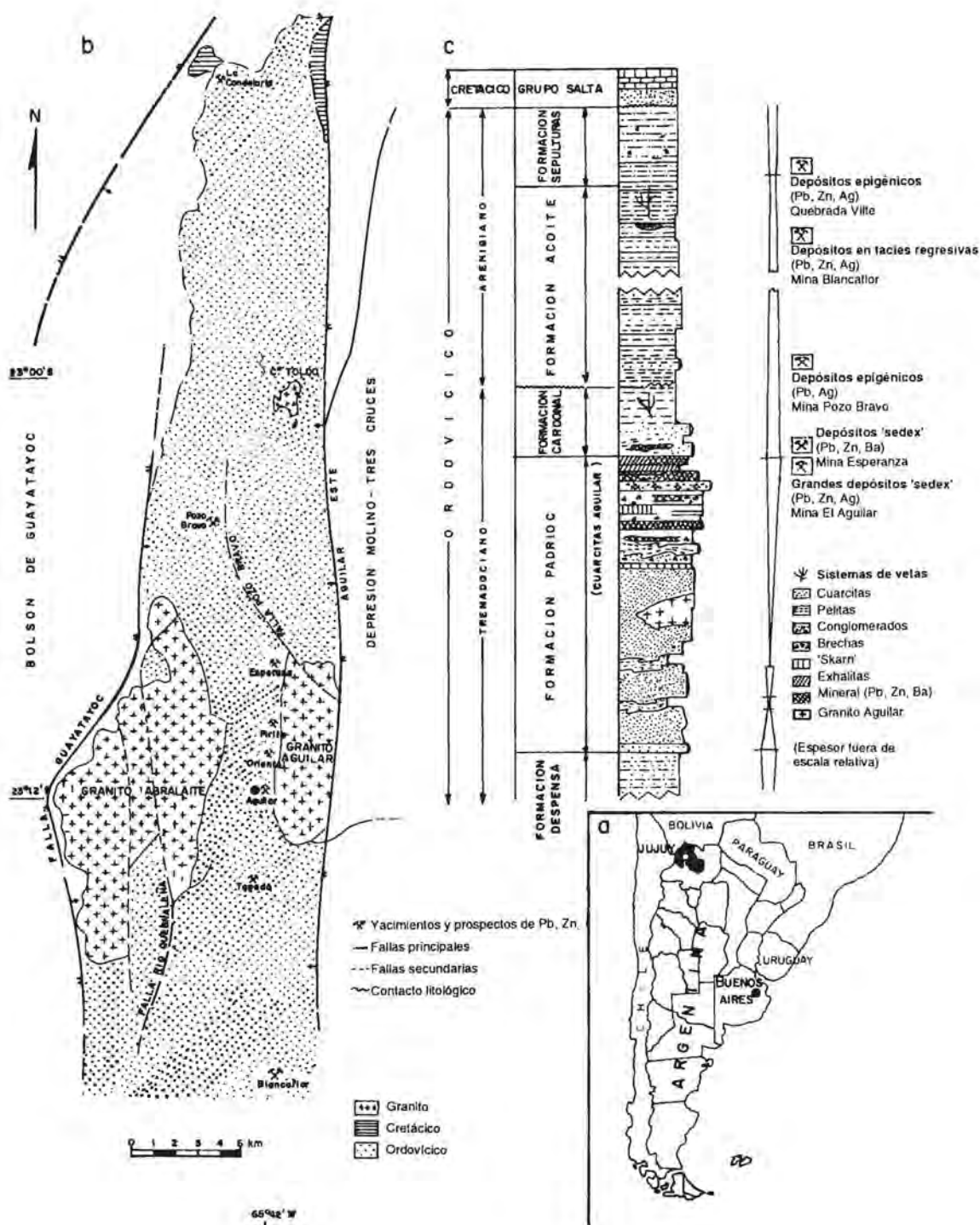
FIG. 1. a- Mapa de ubicación geográfica del área estudiada; b- esquema geológico de la sierra de Aguilar, Jujuy, Argentina; c- columna estratigráfica simplificada, con énfasis en el Paleozoico de la sierra de Aguilar y con la posición de sus yacimientos de plomo y zinc.
