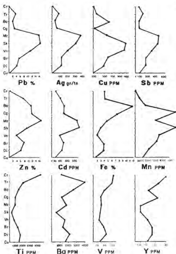
Cuadro 1. Reúne los elementos de filiación sedimentaria-exhalativa introducidos en la Formación Padrioc durante el Tremadociano inferior. Los ocho diagramas iniciales (Pb, Ag, Cu, Sb, Zn, Cd, Fe y Mn) son elementos que se incorporan mayoritariamente en los sucesos principales de emisión hidrotermal y muestran una notable cohesión paragenética frente al ensamble mineral de las menas. Los cuatro últimos diagramas (Ti, Ba, V, Y) e inclusive el Fe, son elementos que tienden a concentrarse con las emisiones finales, al término del episodio metalogénico.
