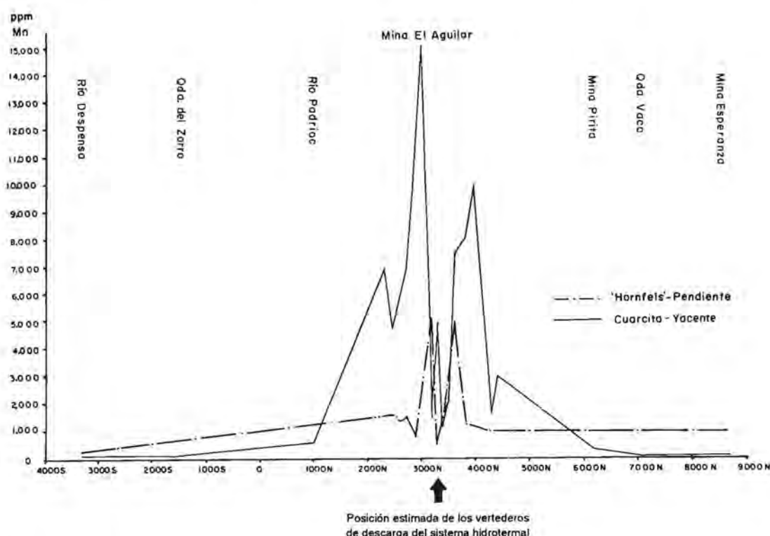
FIG. 6. Perfil geoquímico longitudinal norte-sur, sobre el flanco oriental de la sierra de Aguilar, muestra los contenidos de manganeso de la Formación Padrioc, entre el río Despensa y la mina Esperanza. Las curvas representan dos líneas de muestreo ubicadas en el piso (cuarcitas) y en el techo (corneanas), respectivamente, de la unidad estratigráfica mineralizada en la mina El Aguilar. Su diseño ilustra la extensión del halo de manganeso en el fondo marino del Tremadociano inferior. Se indica la localización estimada de los vertederos del sistema hidrotermal, en posición coincidente con otras evidencias complementarias.
